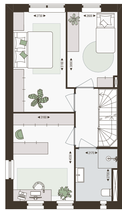
1e verdieping 1:100
