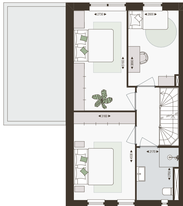
1e verdieping 1:100
