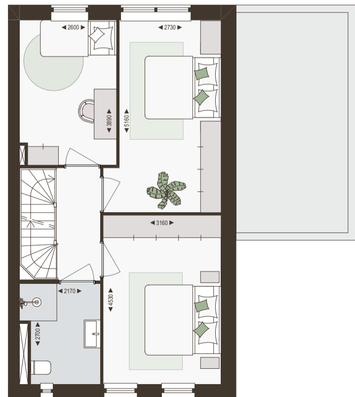
1e verdieping 1:100
