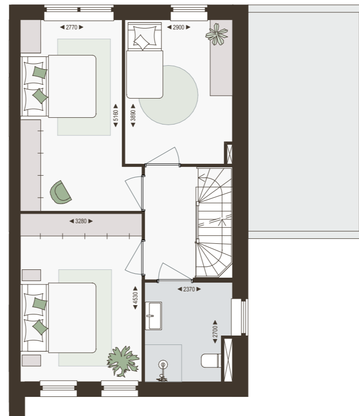
1e verdieping 1:100
