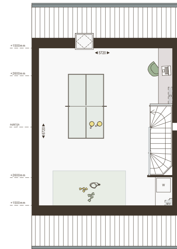
2e verdieping 1:100
