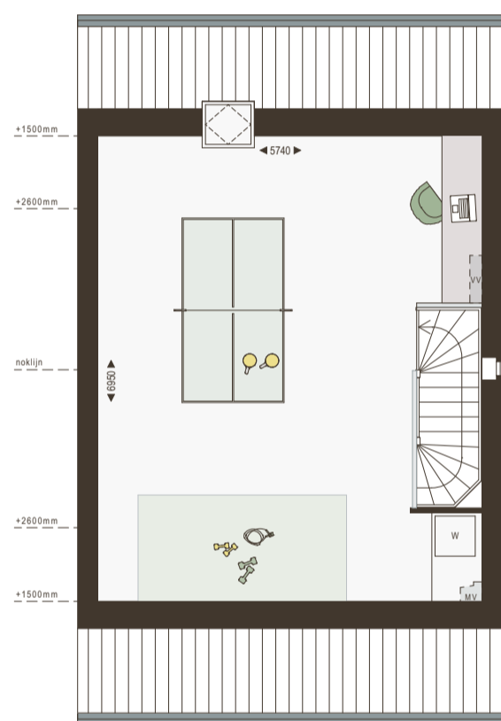
2e verdieping 1:100
