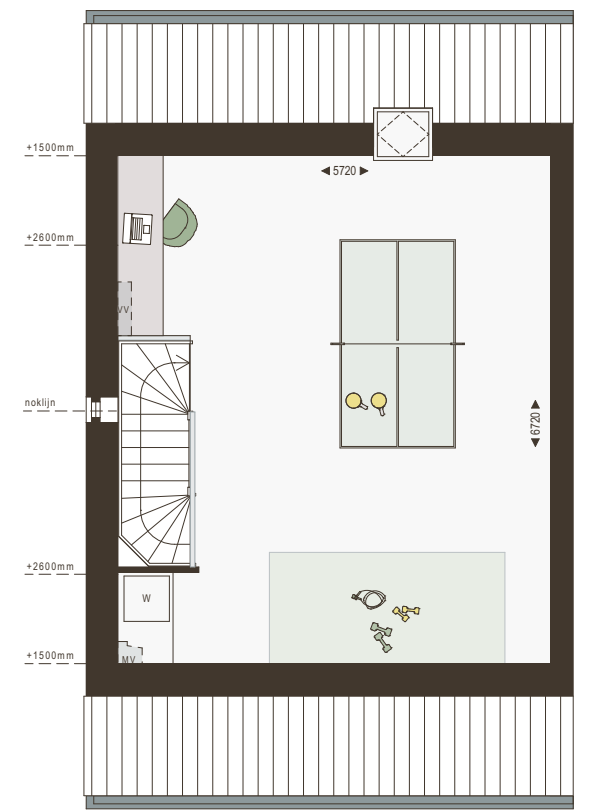
2e verdieping 1:100
