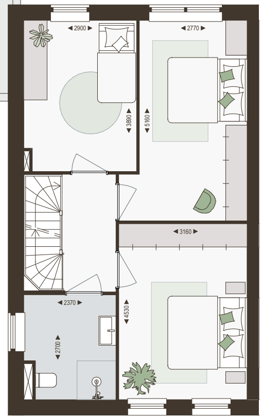
1e verdieping 1:100
