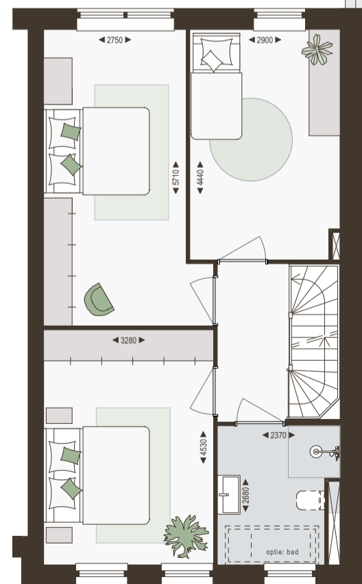
1e verdieping 1:100
