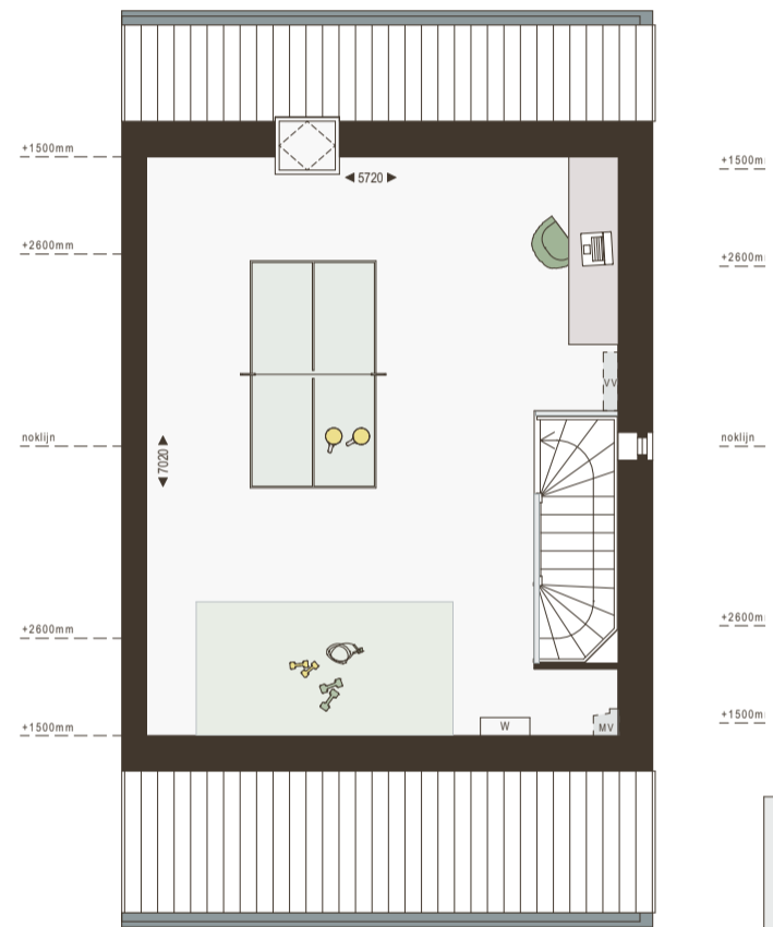
2e verdieping 1:100
