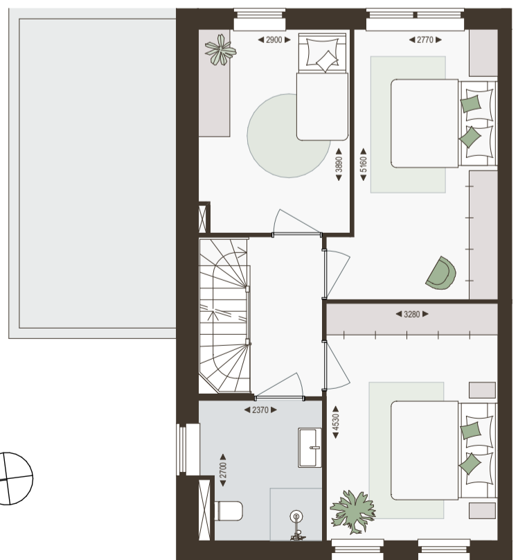
1e verdieping 1:100
