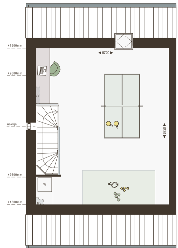
2e verdieping 1:100
